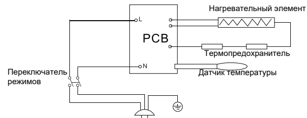
Рис. 2 Электрическая схема
